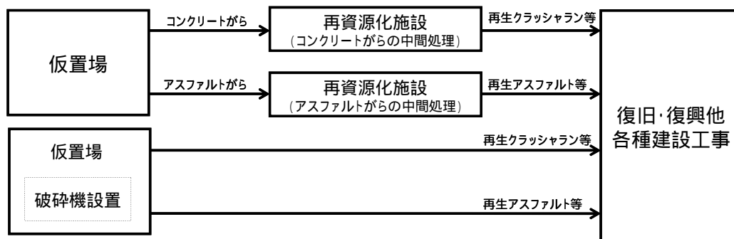
図1 コンクリート及びアスファルトの処理フロー
